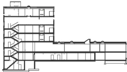
Längsschnitt Hauptgebäude
