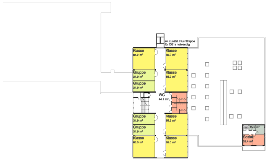
1.Obergeschoss
