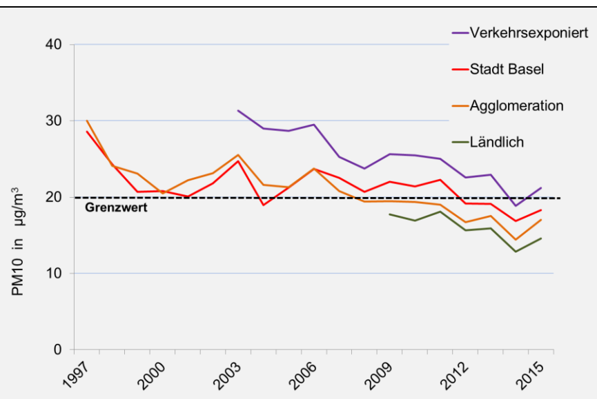
Abb. 12: Entwicklung der PM10-Jahresmittelwerte von 1997 bis 2015
