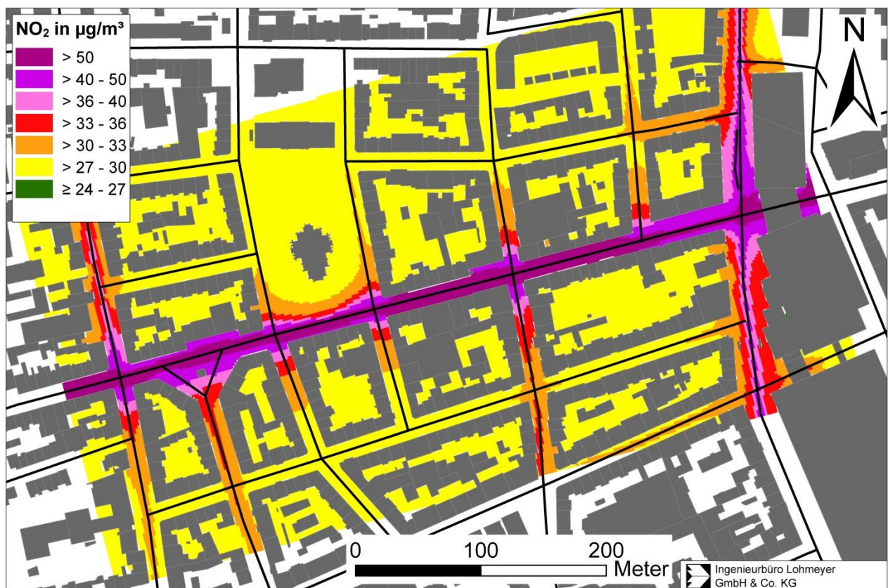
Abb. 39: \text{NO}_2 -Jahresmittelwerte im 2015 an der Feldbergstrasse unter Berücksichtigung Gebäudestruktur
