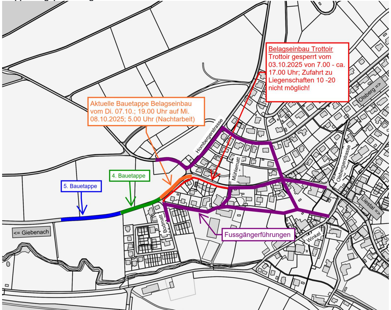
Etappierungsplan Belagseinbau 2025
