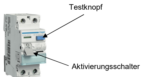
FI-Schutzschalter
