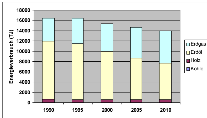
Abb. 4-1: Trendentwicklung Endenergieverbrauch der Feuerungsanlagen im Bereich Haushalte/ Gewerbe/ Dienstleistungen in den Kantonen BS und BL
