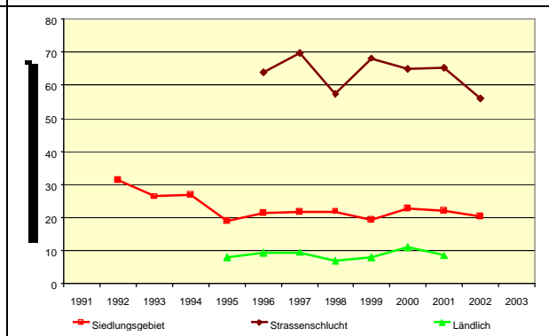
Abb. 4-45: Ozonfördernde VOC - Entwicklung Jahresmittelwerte 1992 - 2002
