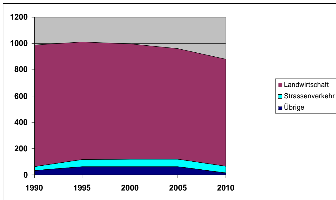
Abb. 4-12: NH_3 -Emissionen der Kantone BS und BL 1990-2010 (Tonnen/Jahr)
