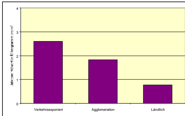
Abb. 4-42: Benzol - Jahresmittelwerte 2000-2002
