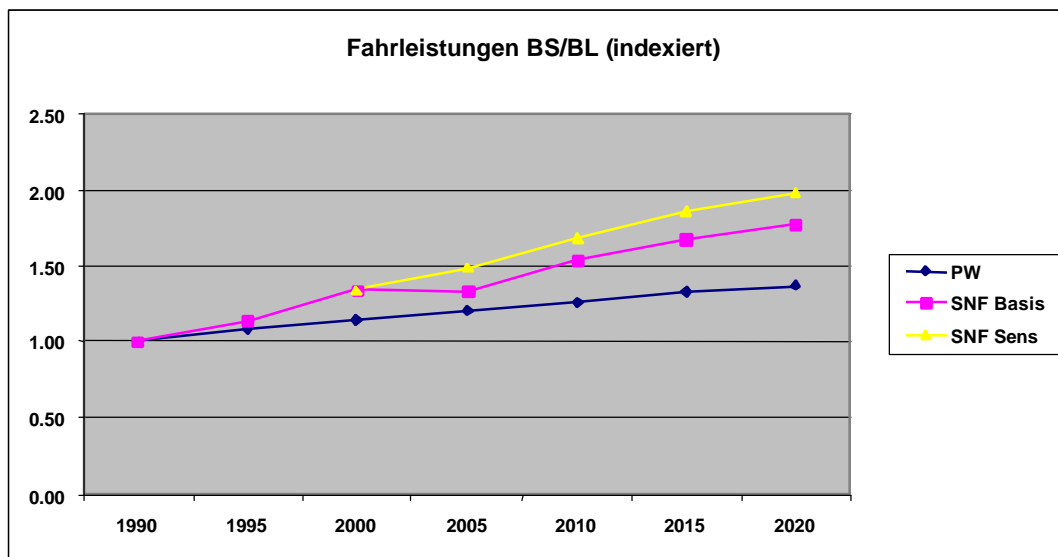
Abb. 4-2: Entwicklung der Fahrleistungen des Strassenverkehrs in den Kantonen BS und BL PW: Personenwagen SNF Basis: Schwere Nutzfahrzeuge, Trendentwicklung nach Einführung 40t-Limite und LSVA SNF Sens: Schwere Nutzfahrzeuge, Sensitivitätsszenario unter Beibehaltung der 28t-Limite
