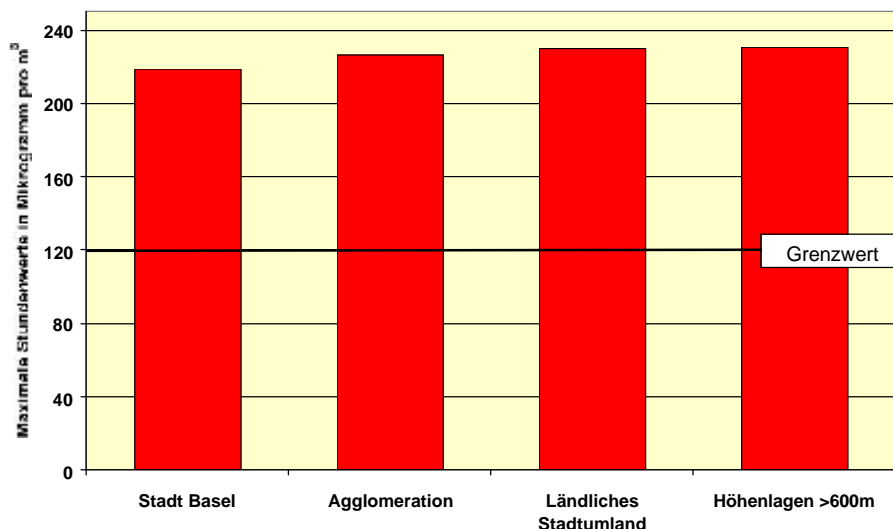
Abb. 4-34: Ozon - Maximalwerte 2003
