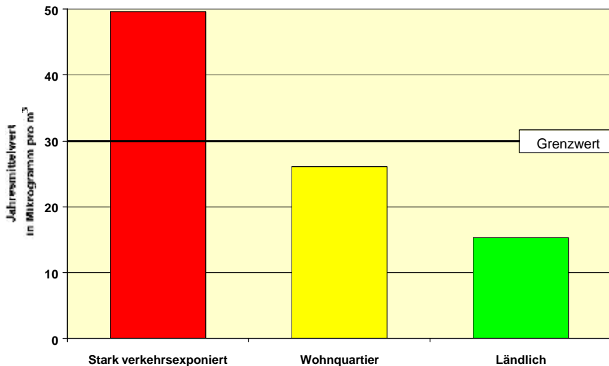
Abb. 4-23: Stickstoffdioxid - Jahresmittelwerte 2003
