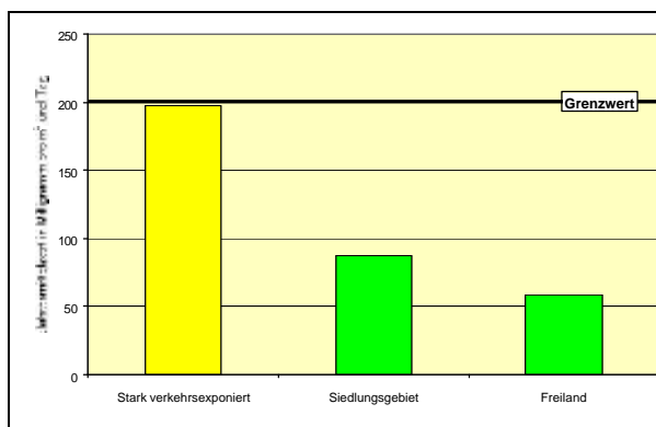
Abb. 4-50: Staubniederschlag - Jahresmittelwerte 1998
