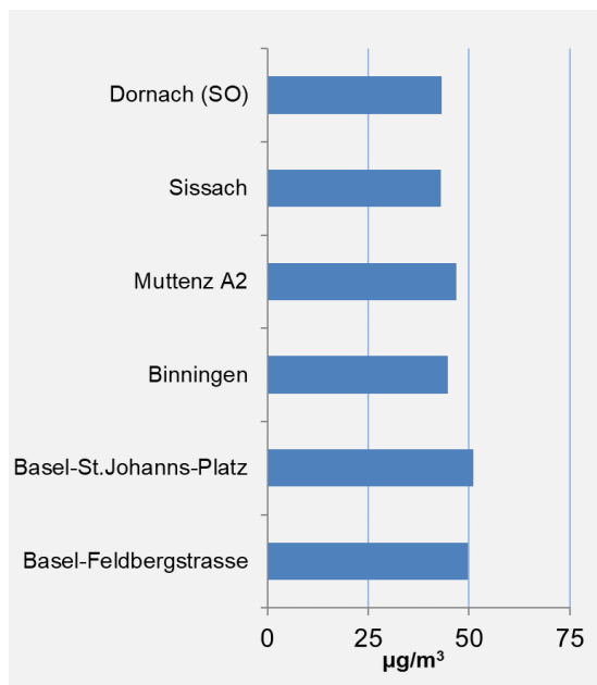
Abb. 12: Maximale Tageswerte im 2023
