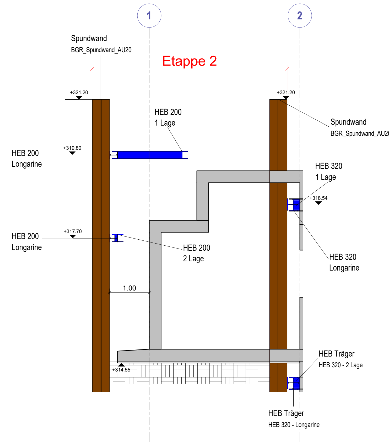
Schnitt A4 M 1 : 50
